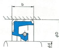
大径SB型
