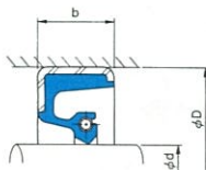
SBB型
