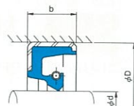
大径SB型
