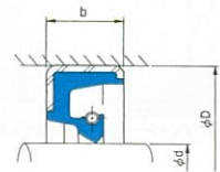
大径SB型
